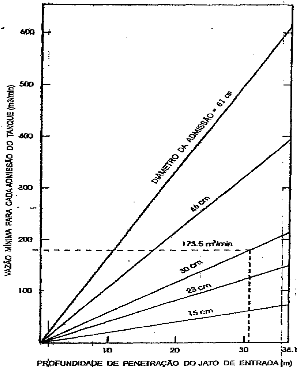
Figura 7-1. Vazão mínima em função da profundidade de penetração do jato A profundidade de penetração do jato deverá ser comparada com a altura do tanque.
