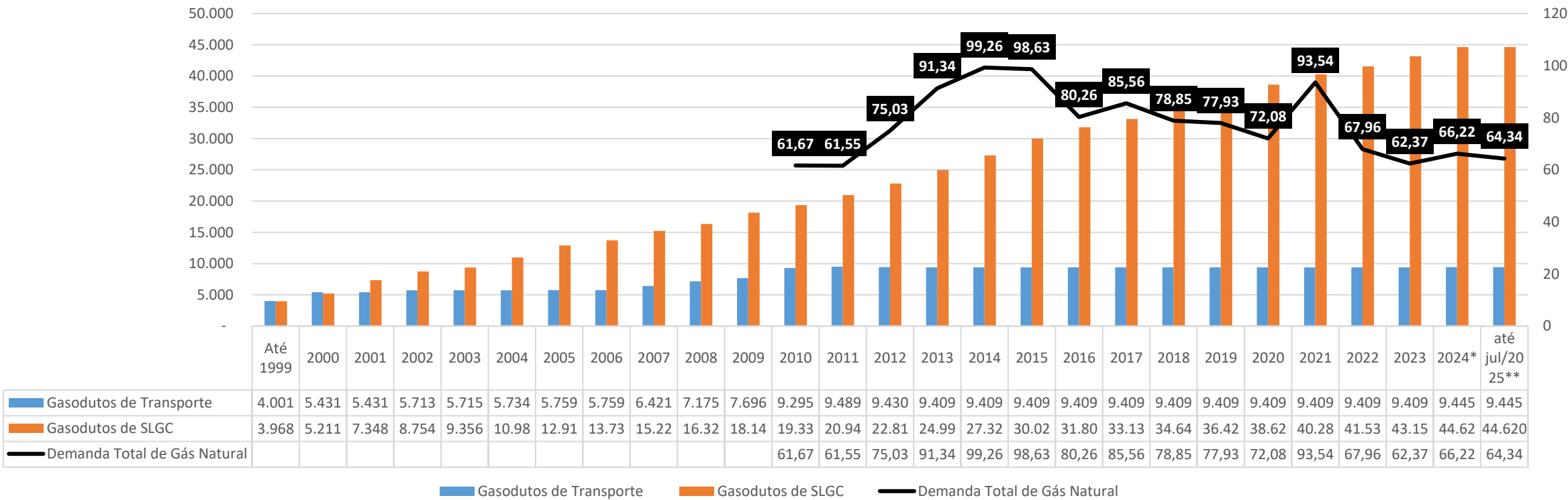
Demanda Total de Gás Natural Nacional vs Extensão de Gasodutos de Transporte e de Serviço Local de Gás Canalizado
