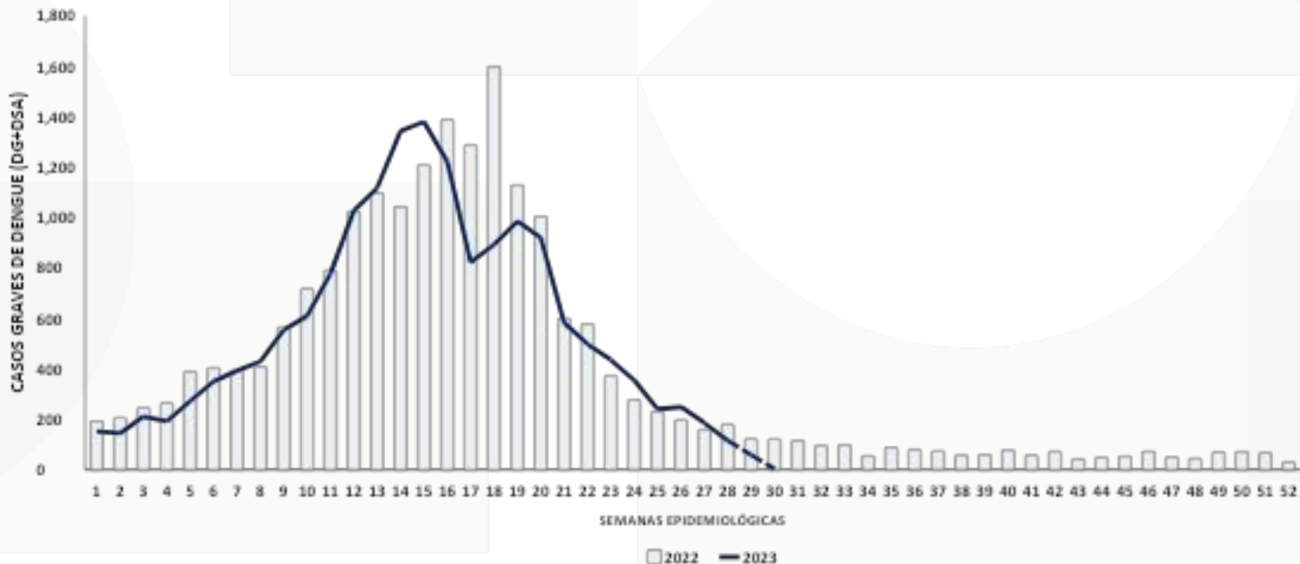
CURVA EPIDÊMICA DE CASOS GRAVES DE DENGUE E DENGUE COM SINAIS DE ALARME (DG+DSA) – 2022 E 2023
