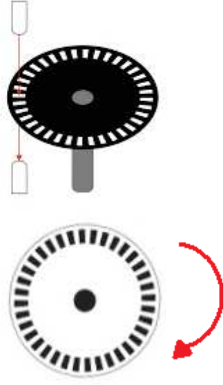
Transdutor óptico
